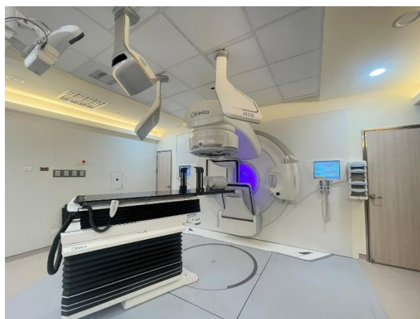
光子治療直線加速器
